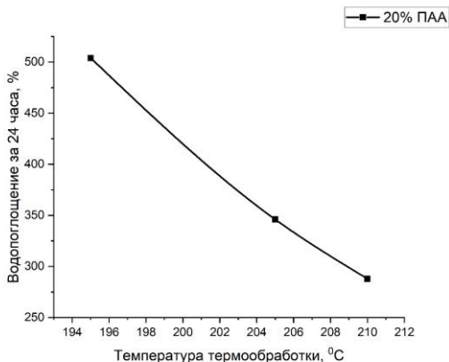
Рисунок 3. Зависимость водопоглощения образцов от температуры термообработки
