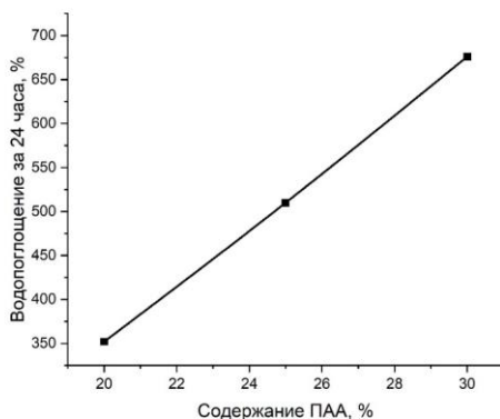
Рисунок 4. Зависимость водопоглощения от содержания ПАА
