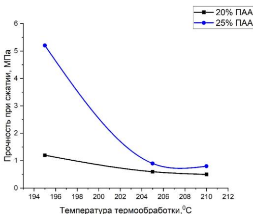
Рисунок 2. Зависимость прочности образцов при сжатии от температуры термообработки
