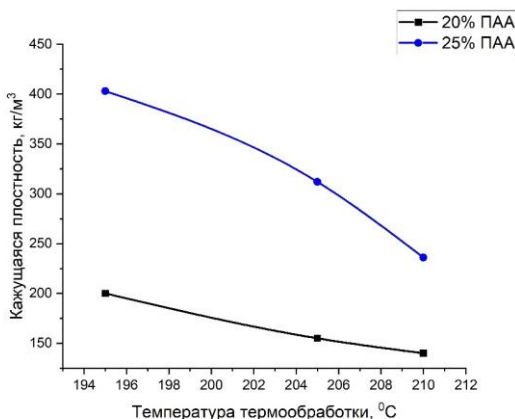
Рисунок 1. Зависимость кажущейся плотности образцов от температуры термообработки
